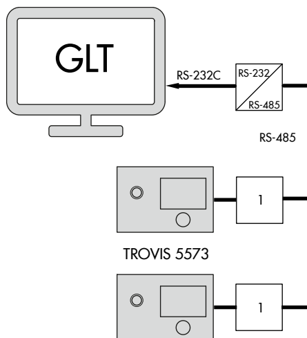
Bild 17: Netzaufbau
