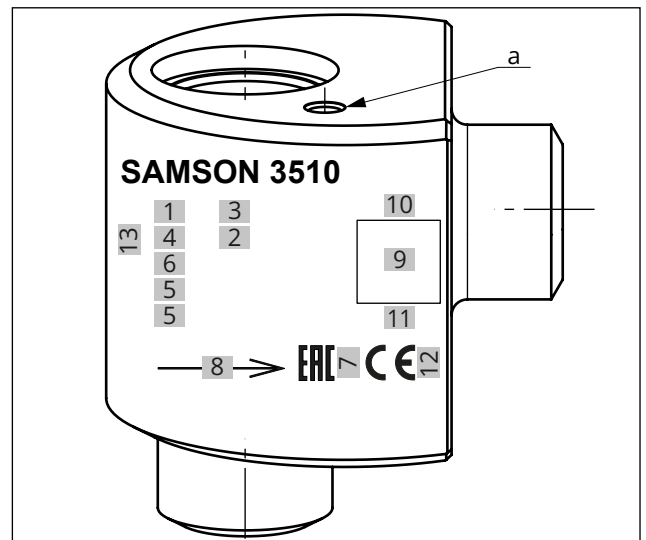
Fig. 4 : Marquage de la vanne à passage équerre · Corps rond
