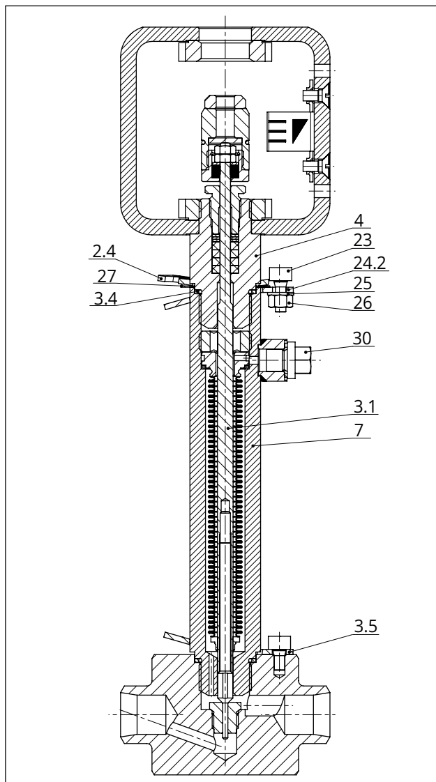
Fig. 11 : Type 3510 avec soufflet et raccord de contrôle
