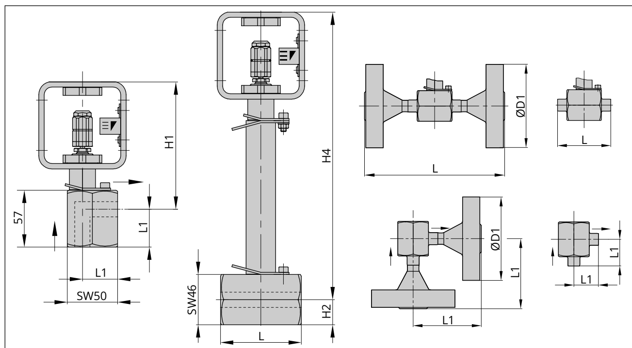
Fig. 8 : de gauche à droite : vanne à passage équerre avec taraudage, vanne à passage droit avec taraudage et soufflet/pièce d'isolement, exécution du corps avec raccord à brides, exécution du corps avec embouts à souder
