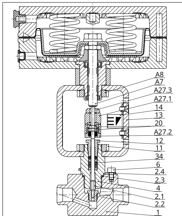
Fig. 9 : Vanne microdébit type 3510 en tant que vanne à passage droit avec servomoteur pneumatique type 3271
