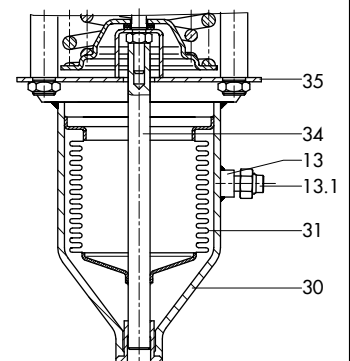
波纹管执行机构： 2 至 6 bar · 5 至 10 bar
