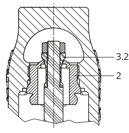
适用于小流量的阀门 K_{VS} \leq 4 ：不带平衡波纹管
