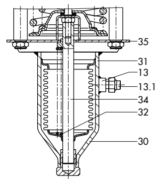
波纹管执行机构： 10 至 22 bar · 20 至 28 bar
