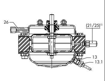
带两个高压灭菌器调节阀 膜片的膜片执行机构（膜片执行机构接头概览）
