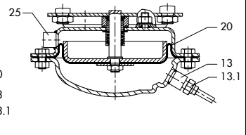
带泄漏管接头的膜片执行机构
