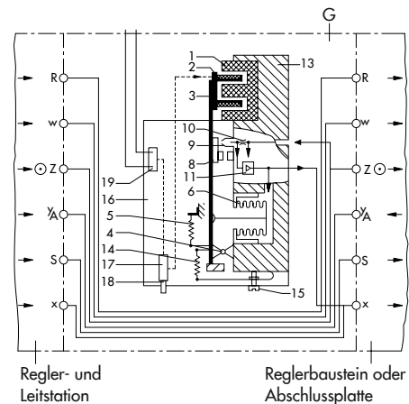
Zusatzbaustein Typ 3424-2... (i/p-Umformer)
