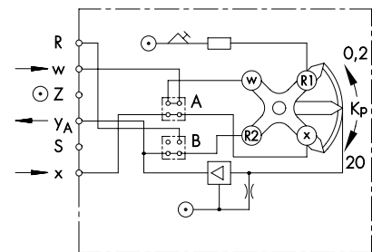
PI-Reglerbaustein Typ 3423-2
