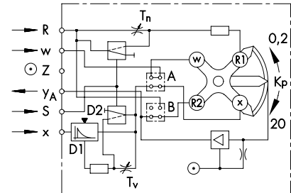
PID-Reglerbaustein Typ 3423-3
