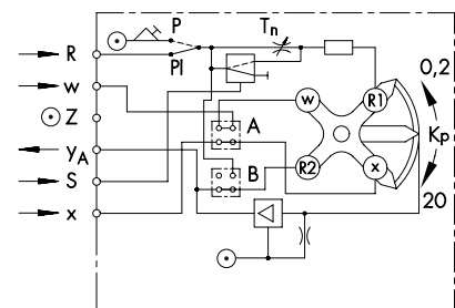
P/PI-Reglerbaustein Typ 3423-5
