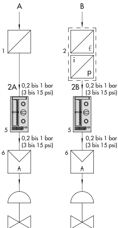
Bild 2: Instrumentierung mit Leitgeräten Typ 3427 oder Leitstationen Typ 3422 und getrennten Warten- oder Feldreglern Typ 3425
