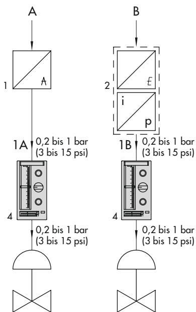
Bild 1: Instrumentierung mit Schalttafeleinbau-Reglern Typ 3421
