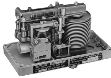
Messumformer Typ 3804-1, Normalausführung
