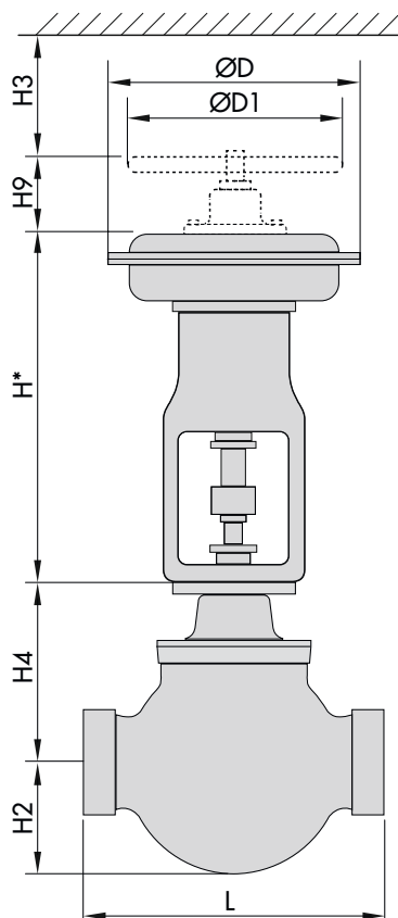
Durchgangsventil Typ 3595 mit pneumatischem Antrieb 3276 Gehäuse mit Anschweißenden oder Vorschuhenden
